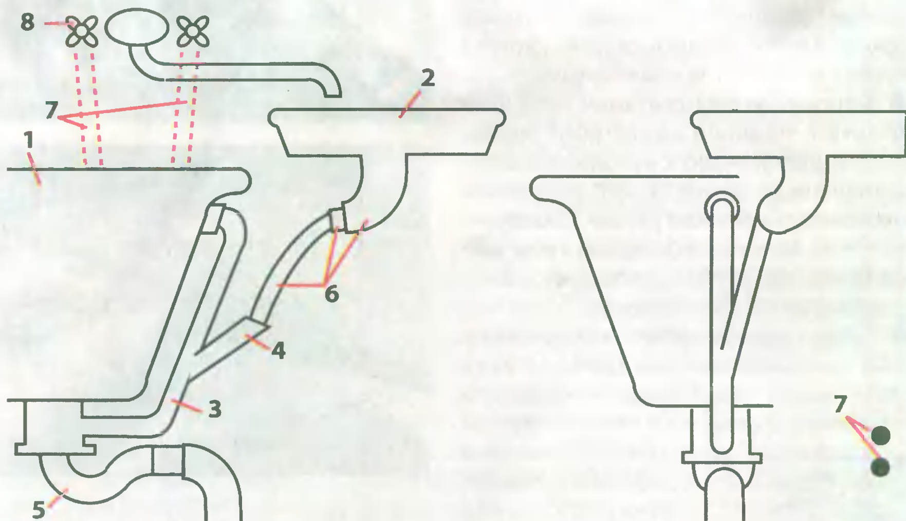
Рис. 2 Технологическая схема
