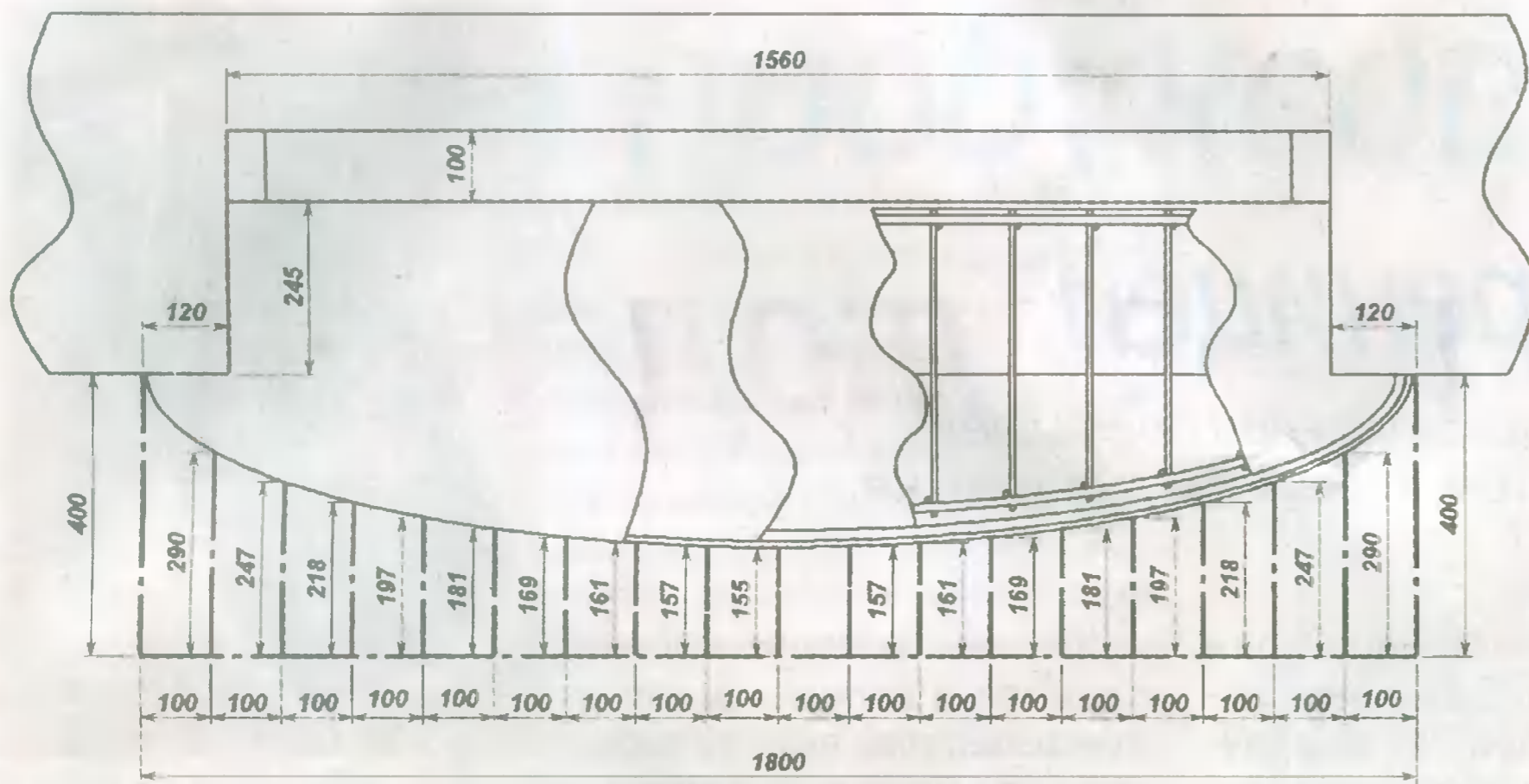
Рис. 3 Чертеж арматурного каркаса
