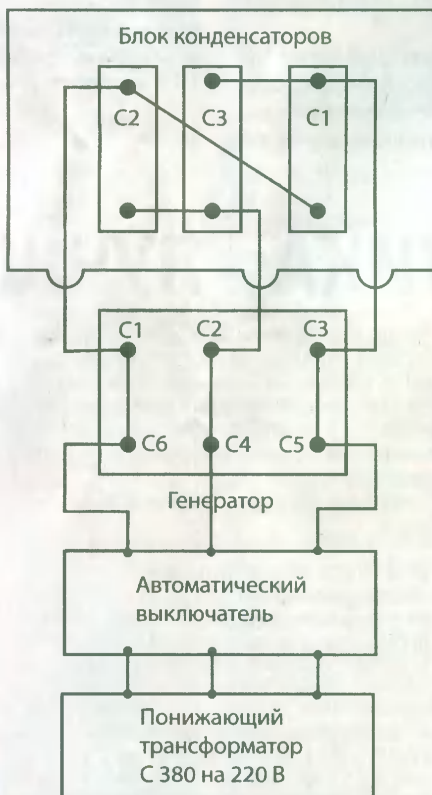
Рис. 2 Монтажная схема
