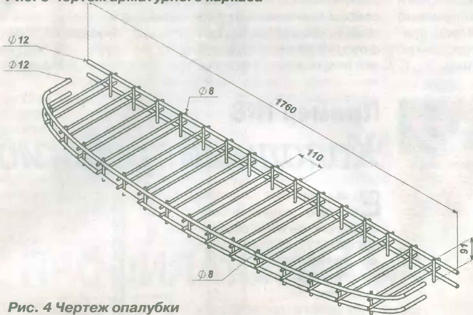
Рис. 3 Чертеж арматурного каркаса
