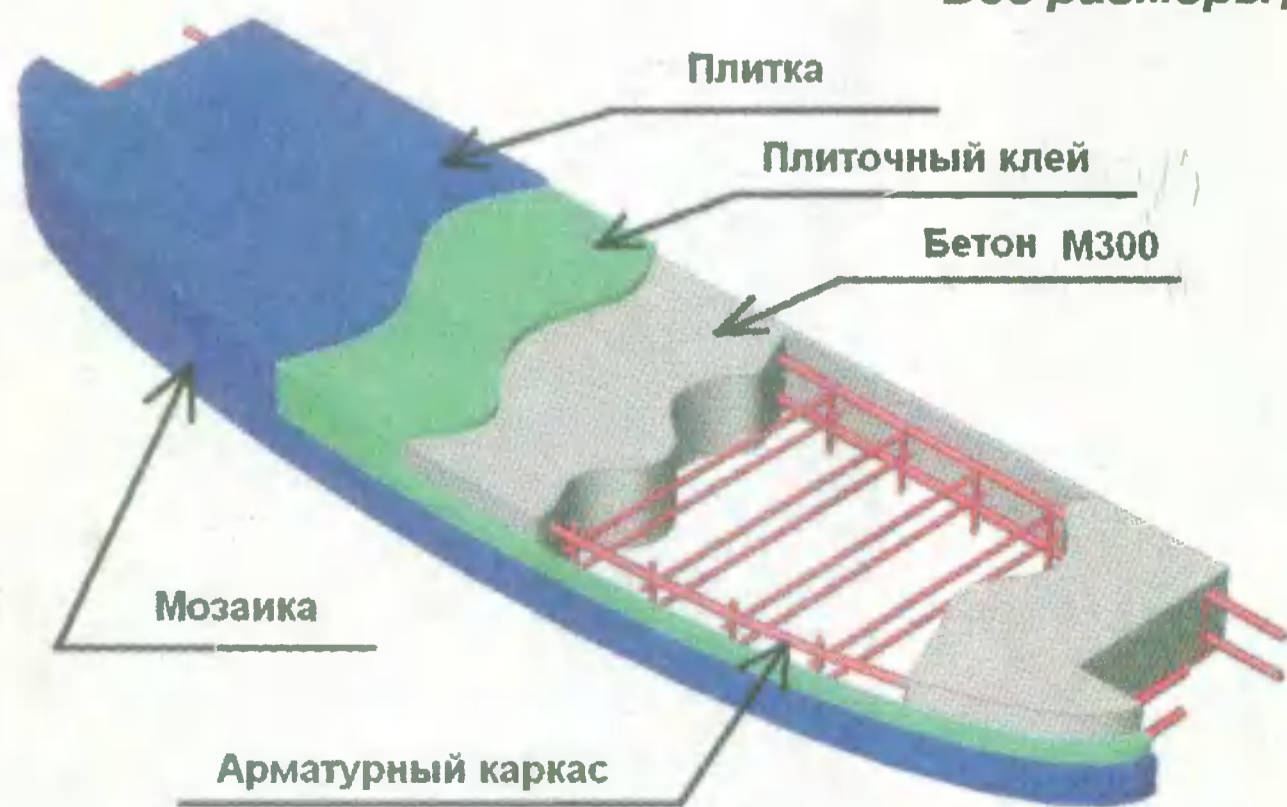
Рис. 1 Структура подоконников
